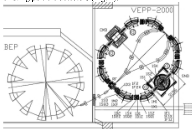
Fig. 1. The VEPP-2000 collider layout.
