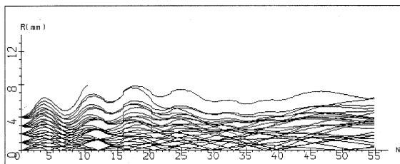
Рис.3. Радиальные траектории частиц, ускоряемых в ПОС-32
