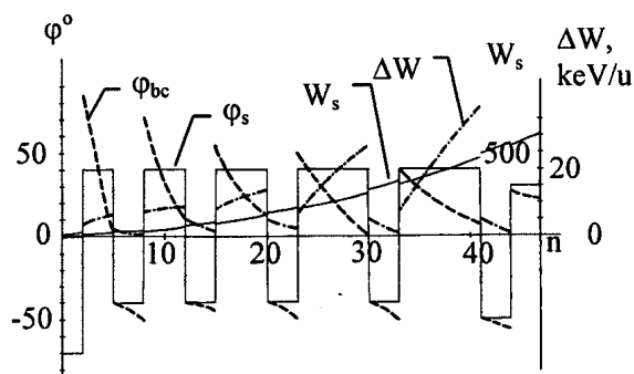
Рис.1. Совмещенный график зависимости фазовых и энергетических характеристик пучка ионов в процессе ускорения на участках структуры ПОС-32
