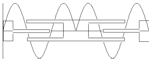
Рис.8. Блок ВЧ-квадруполей для ускорителя протонов среднего диапазона энергий в структуре двухзольных резонаторов CCDTL (coupled-cavity drift tube linac)
