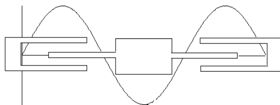
Рис. 6. Схема ВЧ-квадрупольного блока (ВЧКБ) в ускоряющей структуре встречно-штыревого типа
