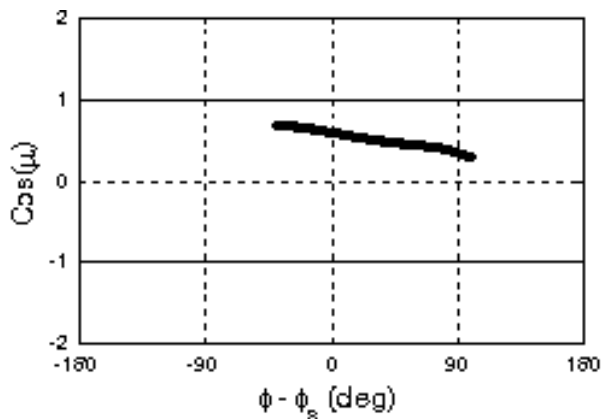
Рис. 5. Косинус набег фазы радиальных колебаний частиц в зависимости от фазы влета в ускоряющефокусирующий период
