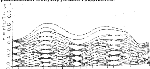
Рис. 7. Траектории радиального движения частиц в структуре начальной части ПОС-46
