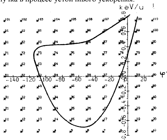
Рис.2. Сепаратриса, определяющая захват инжектируемого пучка в процесс устойчивого ускорения
