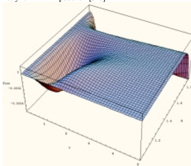
Рис. 4. Поверхность, представляющая зависимость потока частиц в фазовом пространстве от скорости и параметра неэкстенсивности
