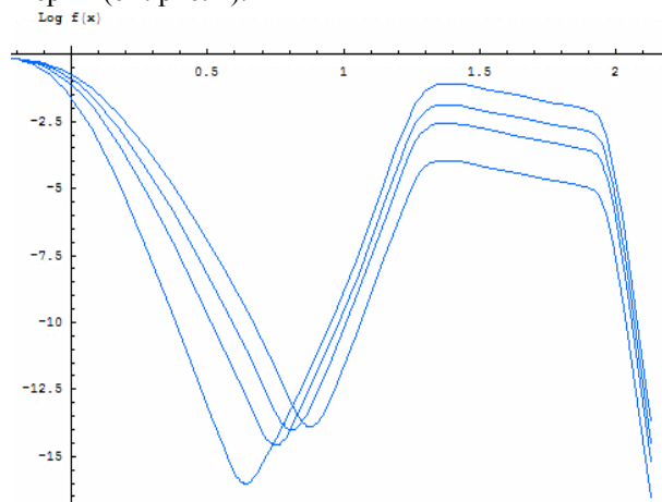
Рис.3. Графики функций распределения в двойном логарифмическом масштабе при T_e=0.1 . Кривые соответствуют P=-1.81, -0.81, -0.4, -0.1
