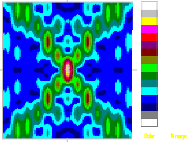
Рис.12. Проекция тела неопределенности ФКМ сигнала (код Баркера)
