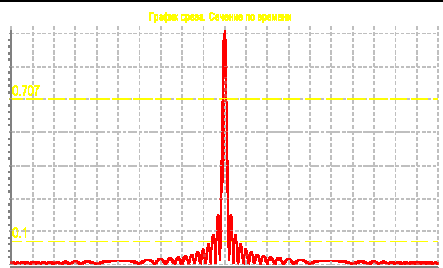
Рис.5. Автокорреляционная функция ЛЧМ сигнала
