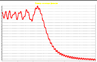
Рис.4. Нормированный амплитудный спектр ЛЧМ сигнала
