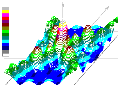
Рис.11. Тело неопределенности ФКМ сигнала (код Баркера)
