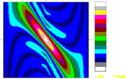
Рис.7. Проекция тела неопределенности ЛЧМ сигнала
