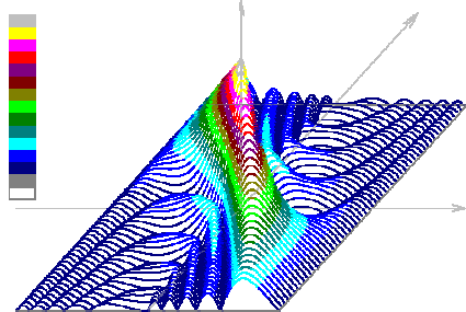
Рис. 6. Тело неопределенности ЛЧМ сигнала
