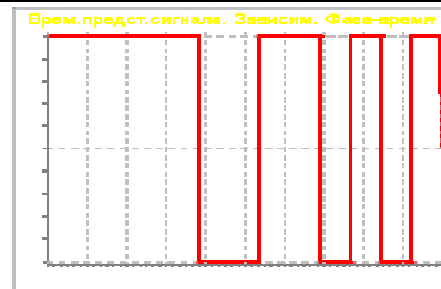
Рис.8. Нормированная зависимость фаза-время для ФКМ сигнала
