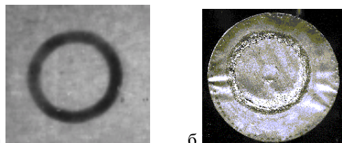
Рис. 6. Автографы пучка: а – обскурграмма пучка, б – след пучка на аноде
